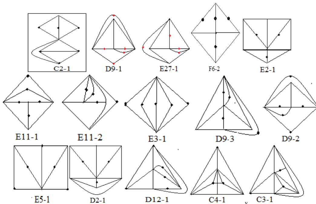
РИС. 5. Наведено графи з виділеними жирним вершинами із множин M з клітковою відстанню 2, де (t_G(M) = 3) \wedge (\theta_G(M) = 1) , мінімальні відносно кліткової довжини 2 показаних жирним точок множин
