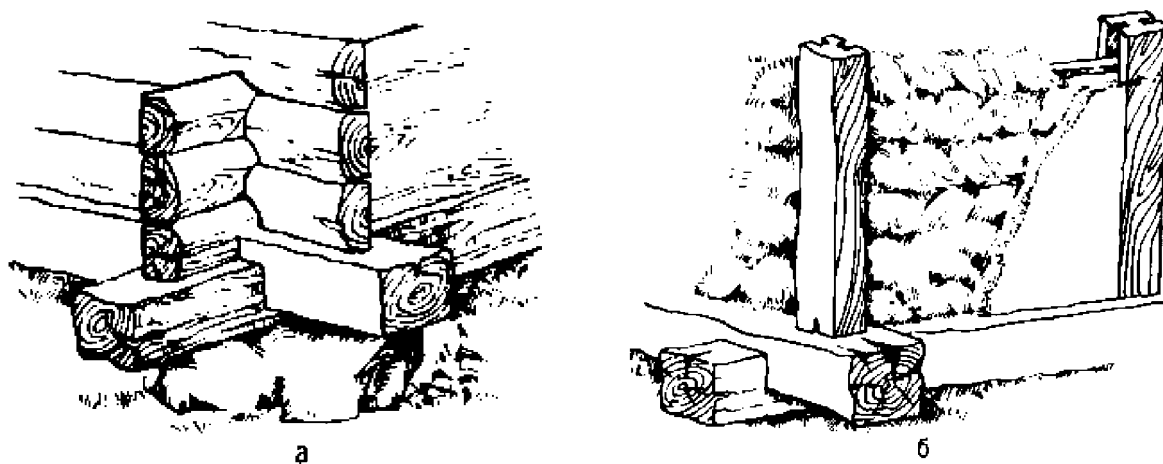
Ил. 1. Зрубна (а) та каркасно-стовпова (б) конструкції стін. За: Українська минувшина [5, с. 21]
