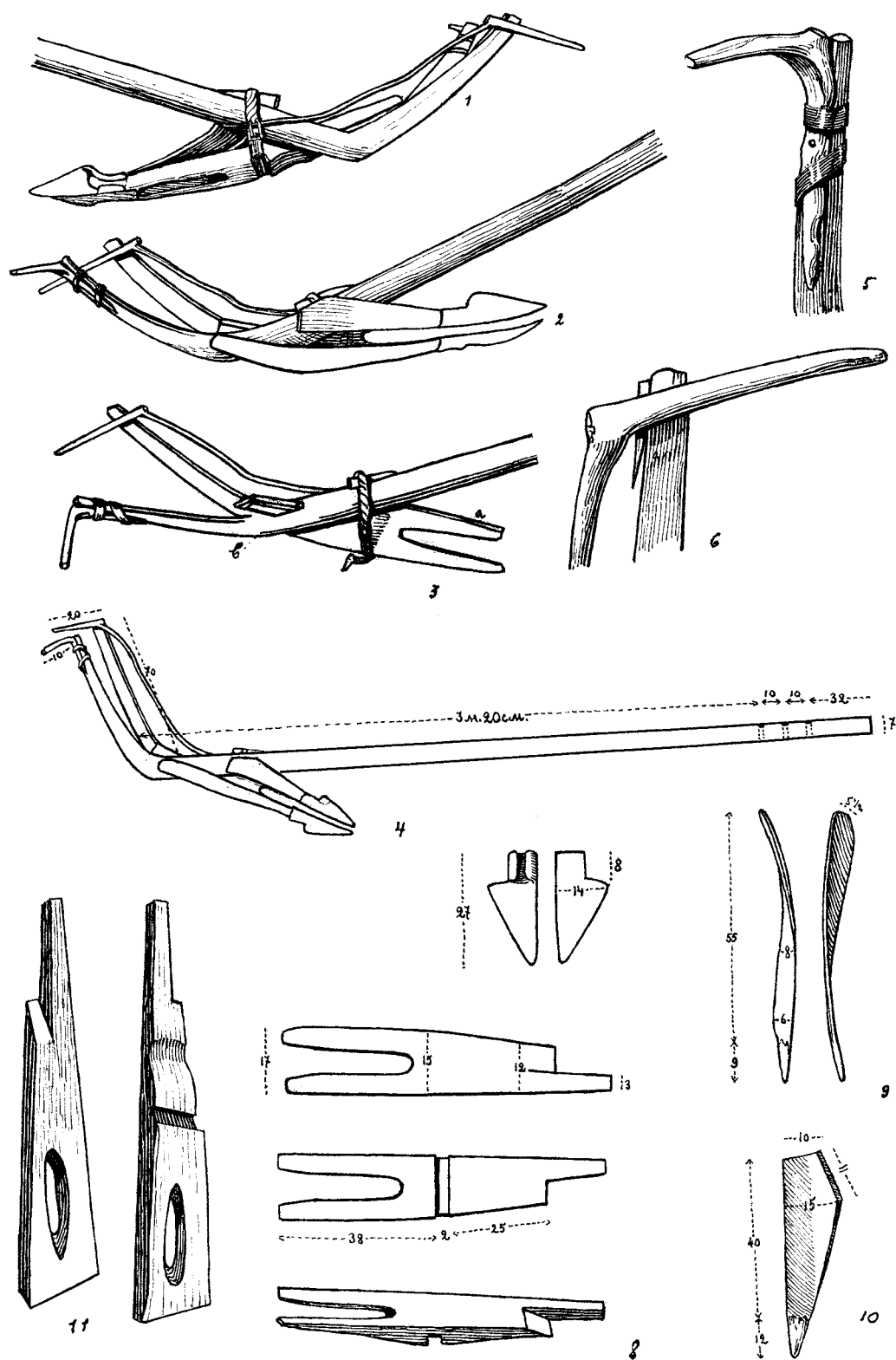
Табл. I. Соха та її деталі.
