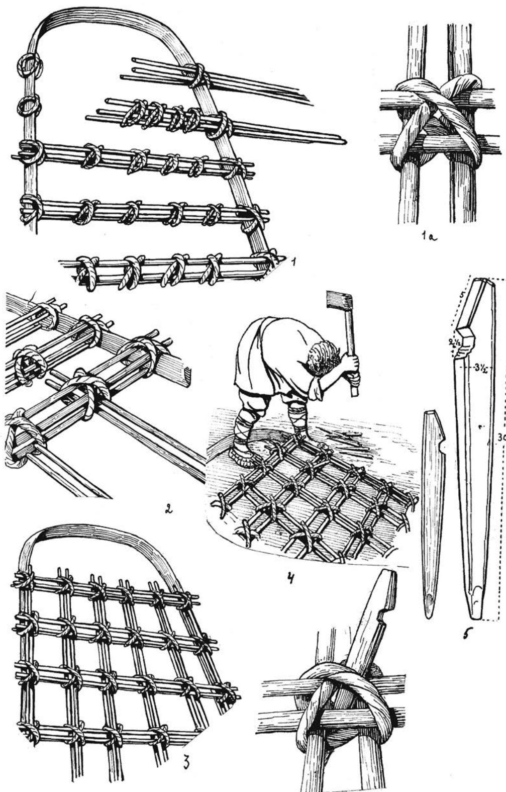
Табл. IV. Складання борони.
