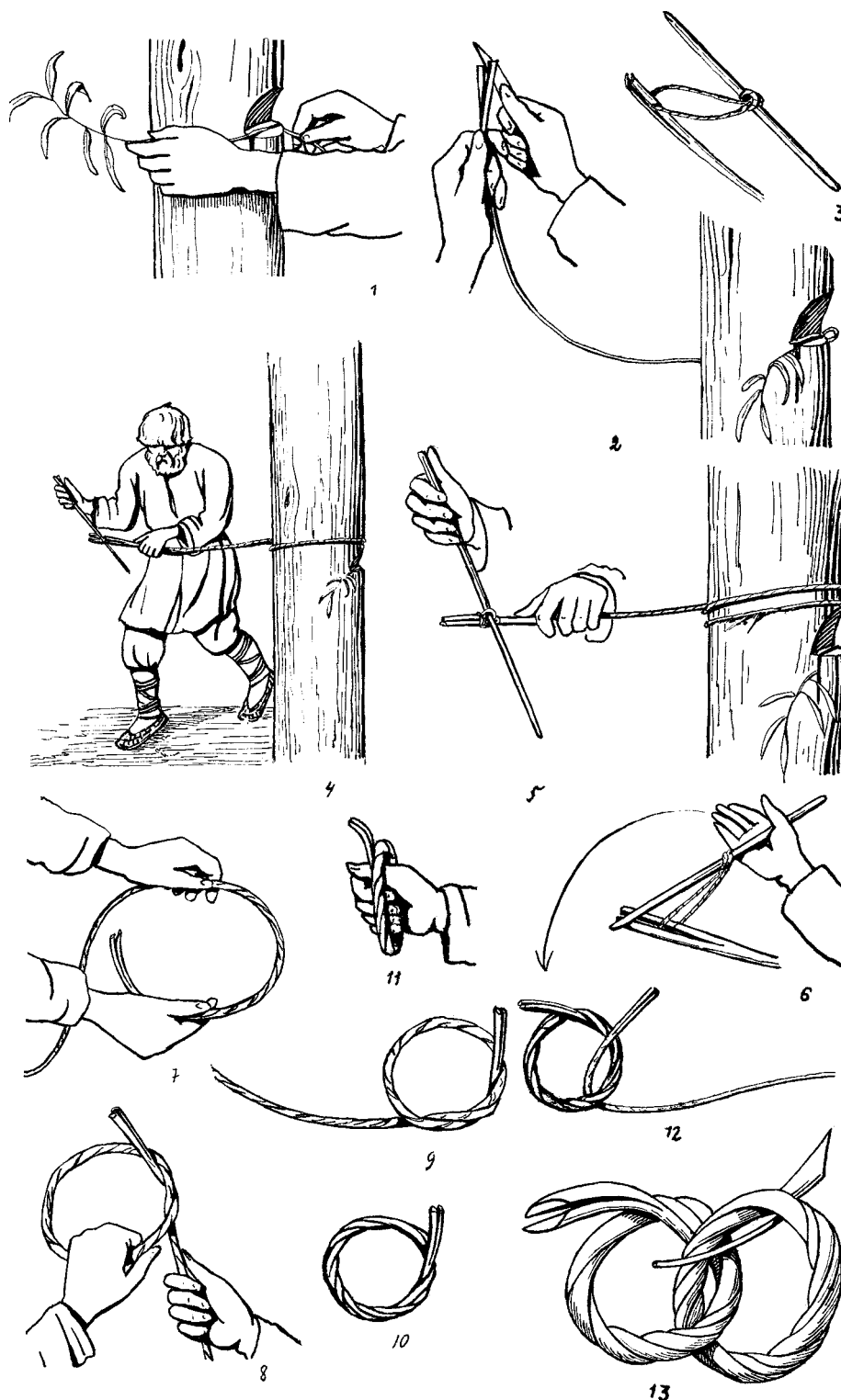
Табл. III. Виготовлення т. зв. колачів.
