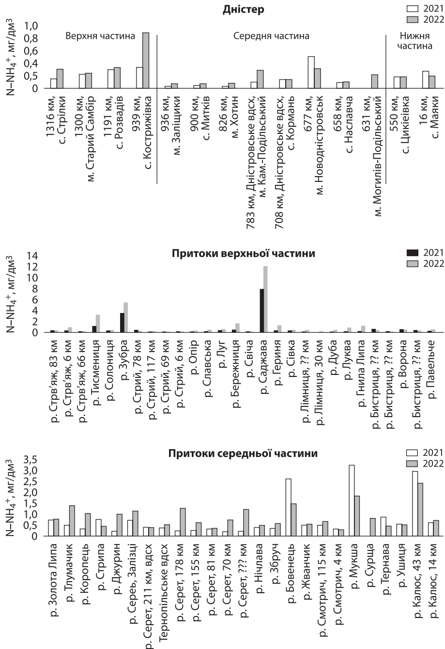
Рис. 8. Співвідношення середніх за рік значень N-NH_4^+ у точках моніторингу: за довжиною р. Дністер; притоків верхньої частини; притоків середньої частини
