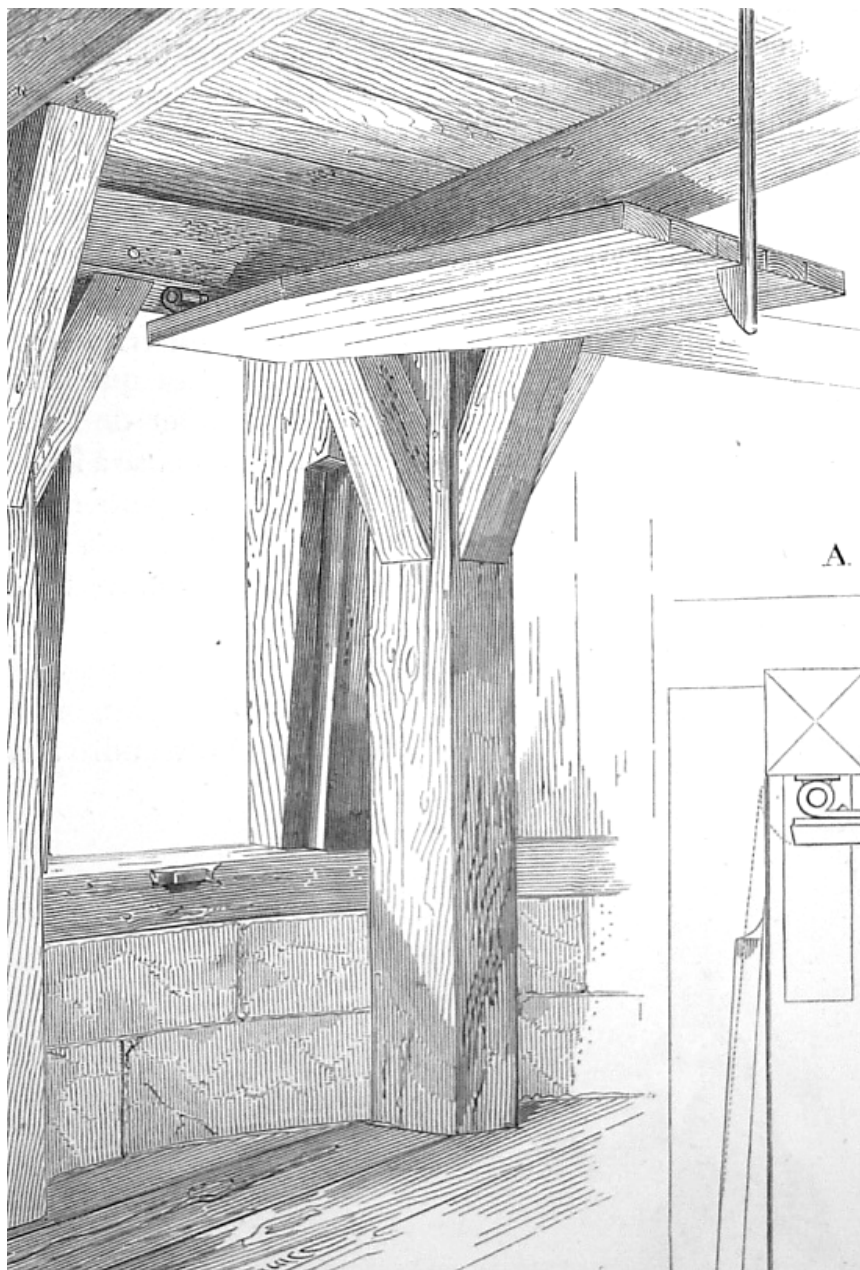
Ил. 7. Один из способов открывания проемов в оборонительных сооружениях. По Виолле-ле-Дюк.
