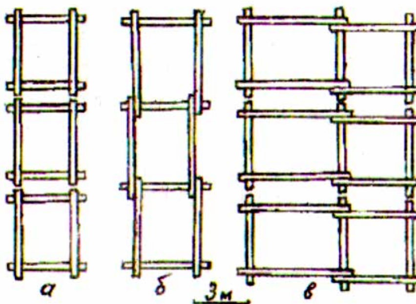
Ил.12. Принципиальные хемы планов срубных клетей. 21 а – цепочка отдельно стоящих стубов; б – цепочка из взаимосвязанных стубов; в – цепочка смешеной конструктивной схемой.
