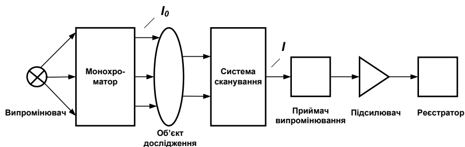
Рис. 2. Структура фотометра
