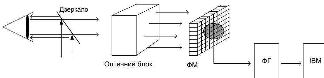
Рис.1 Структурна схема оптико-електронної системи. ФМ – фотоматриця; ФГ – фреймгабер
