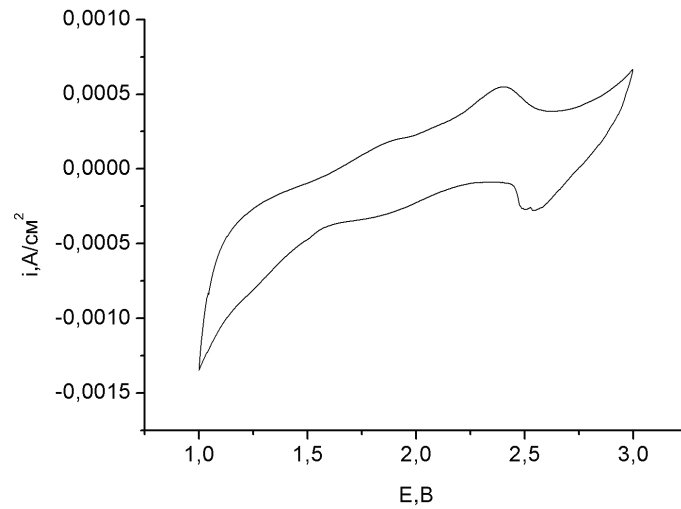
Рис.3. Циклічна потенціодинамічна крива процесу літійової інтеркаляції неосвітленого p - GaSe , виміряна в темряві при швидкості розгортки потенціалу 0,001V/c
