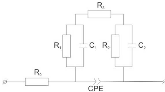
Рис.6. Еквівалентна електрична схема для процесів фотоінтеркаляції- фотодеінтеркаляції
