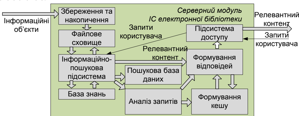
Рис. 2. Концептуальна структура серверного модуля IC Virtual Library
