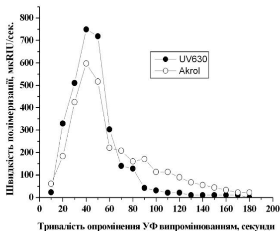
Рис. 5. Залежність швидкості полімеризації від тривалості експозиції ультрафіолетом для двох марок фотополімерних клеїв Akro1-3-360 та UV630.
