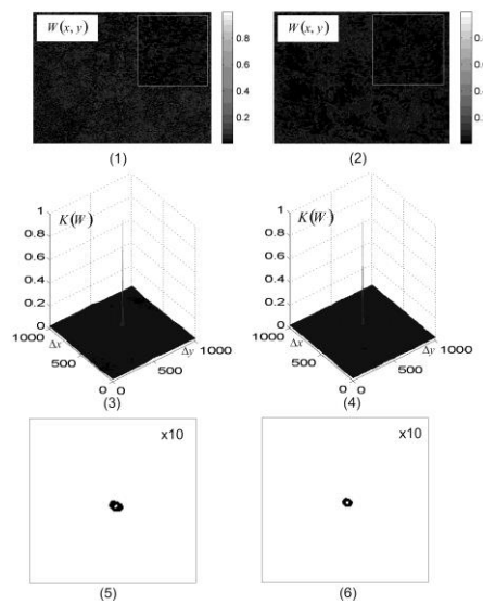
Рис. 1. Координатні розподіли значень W(x, y) (фрагменти (1),(2)), двовірні автокореляційні функції K(W, x, y) (фрагменти (3),(4)) та кореляційні К-контури (фрагменти (5),(6)) гістологічних зрізів біопсії фіброміоми (фрагменти (1),(3),(5)) і аденокарциноми (фрагменти (2),(4),(6))
