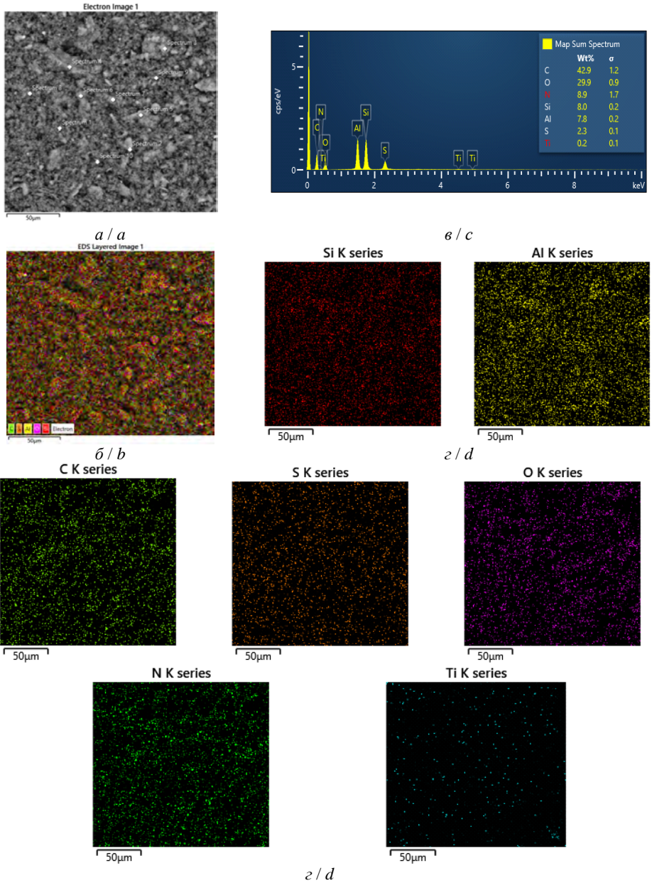
Рис. 6. СЕМ-зображення (а), загальна елементна карта (б), ЕДС-спектр (в) та індивідуальні карти елементів (г) для зразка Цт/ПАН до адсорбції Cr(VI).
