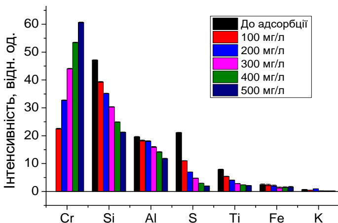
Рис. 10. Вплив концентрації вихідних розчинів Cr(VI) на вміст елементів в адсорбенті Цт/ПАН після адсорбції.
