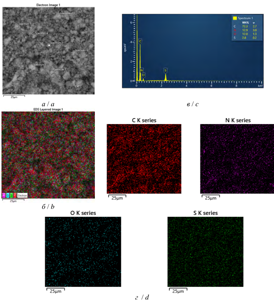
Рис. 4. СЕМ-зображення (а), загальна елементна карта (б), ЕДС-спектр (в) та індивідуальні карти елементів (г) для зразка ПАН до адсорбції Cr(VI).
