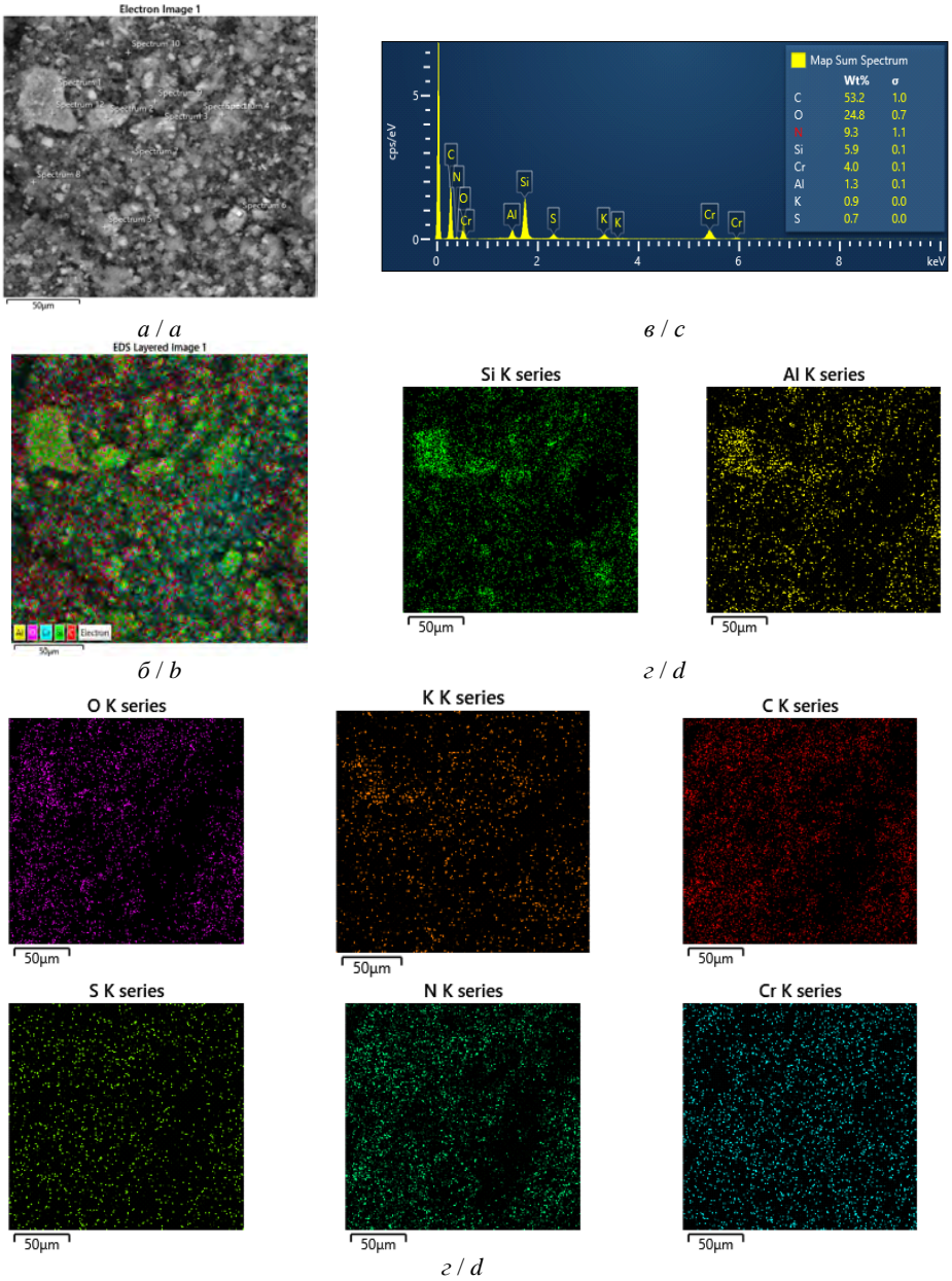
Рис. 9. СЕМ-зображення (а), загальна елементна карта (б), ЕДС-спектр (в) та індивідуальні карти елементів (з) для зразка Цт/ПАН після адсорбції Cr(VI) з розчину з концентрацією 500 мг/л.
