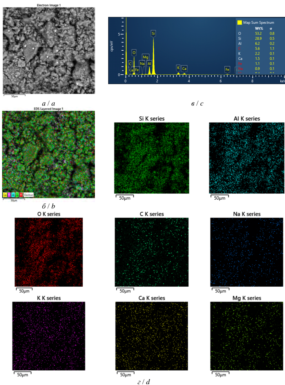
Рис. 2. СЕМ-зображення (а), загальна елементна карта (б), ЕДС-спектр (в) та індивідуальні карти елементів (г) для вихідного зразка Цт.
