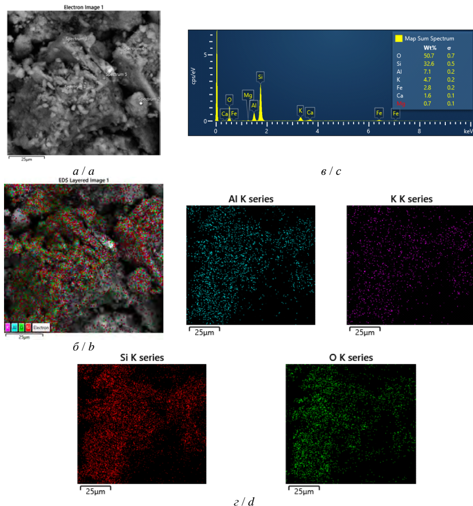
Рис. 3. СЕМ-зображення (а), загальна елементна карта (б), ЕДС-спектр (в) та індивідуальні карти елементів (г) для зразка Цт після адсорбції Cr(VI) з розчину з концентрацією 500 мг/л.
