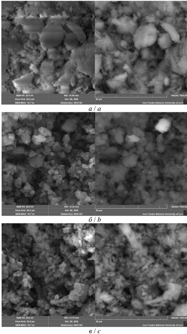
Рис. 1. СЕМ-зображення зразків Цт (а), ПАН (б) та Цт/ПАН (в), отримані у SE (зліва) та BSE (справа) режими. Збільшення у 10700 разів.
