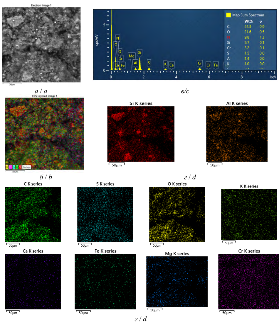
Рис. 8. SEM-зображення (а), загальна елементна карта (б), ЕДС-спектр (в) та індивідуальні карти елементів (г) для зразка Цт/ПАН після адсорбції Cr(VI) з розчину концентрацією 300 мг/л.
