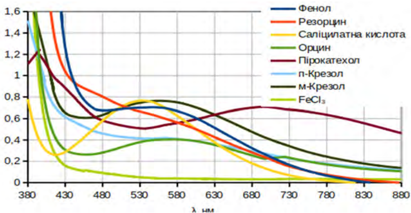
Спектри оптичного поглинання фенольних комплексів \text{Fe}^{3+} при концентраціях фенольних похідних 10^{-5}\text{M} та 10-ти кратному надлишку \text{Fe}^{3+} .
