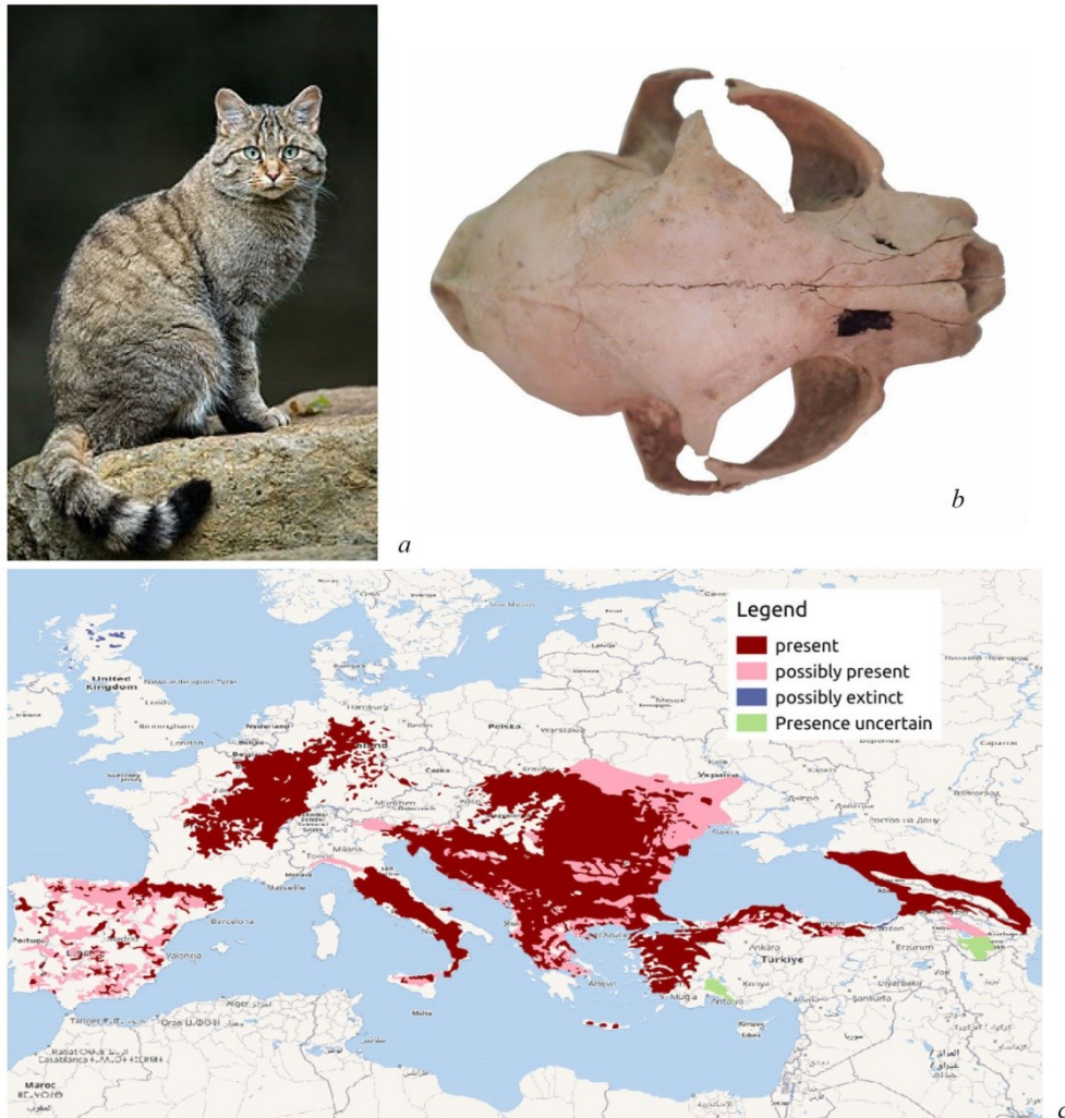
Рис. 2. Кіт лісовий Felis silvestris (s. str.): (a) загальний вигляд тварини (wikimedia.org; User: Lviatour, CC BY-SA 3.0); (b) череп F. silvestris (s. str.) (фото П. Гольдіна); (c) ареал поширення (wikimedia.org; User: BhagyaMani; CC BY-SA 4.0).
