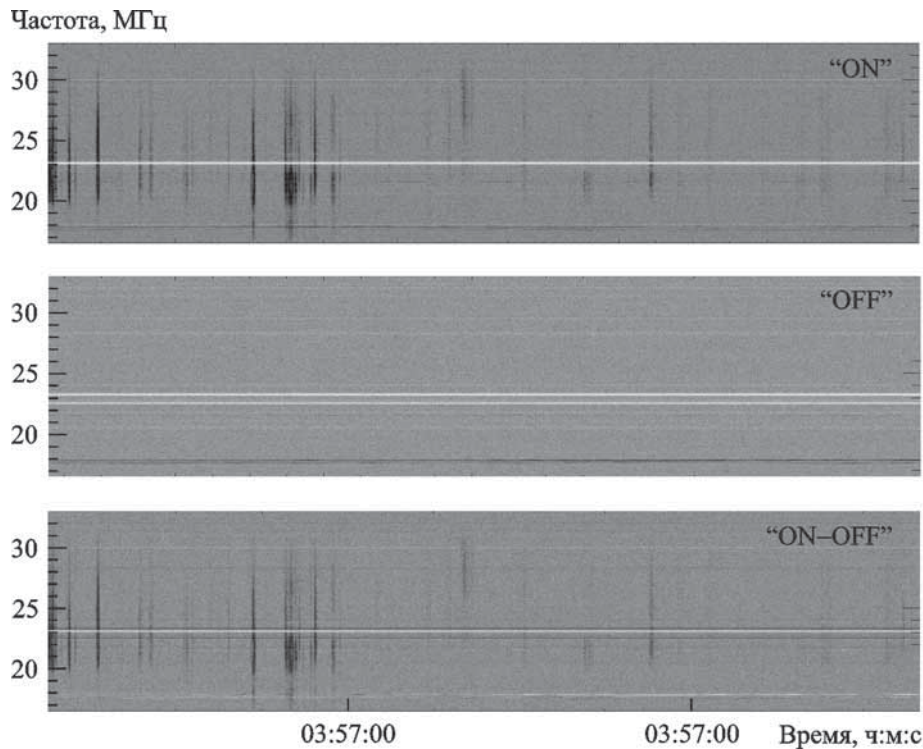
Рис. 1. Модуль кросс-спектра сигналов антенн С–Ю и З–В для “ON” (верхняя панель) и “OFF” (средняя панель) каналов. Нижняя панель – результат вычитания, “ON–OFF”
