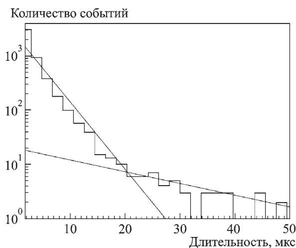
Рис. 4. Гистограмма распределения по длительности микросекундных структур молнии, полученная при временном разрешении 2 мкс. Прямыми показаны аппроксимации функциями вида \exp(-t/t_{ch}) , t_{ch} = 3.5 и 18 мкс
