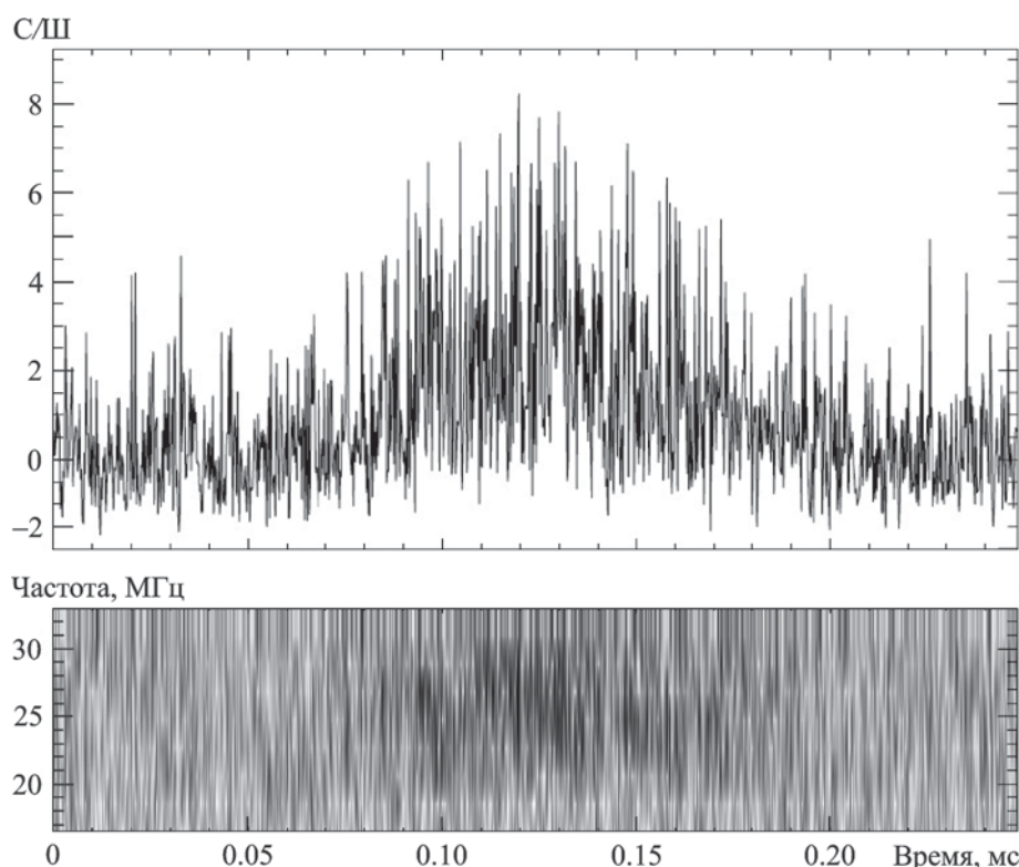
Рис. 6. Профиль сигнала (верхняя панель) и спектрограмма с временным разрешением 500 нс (нижняя панель)
