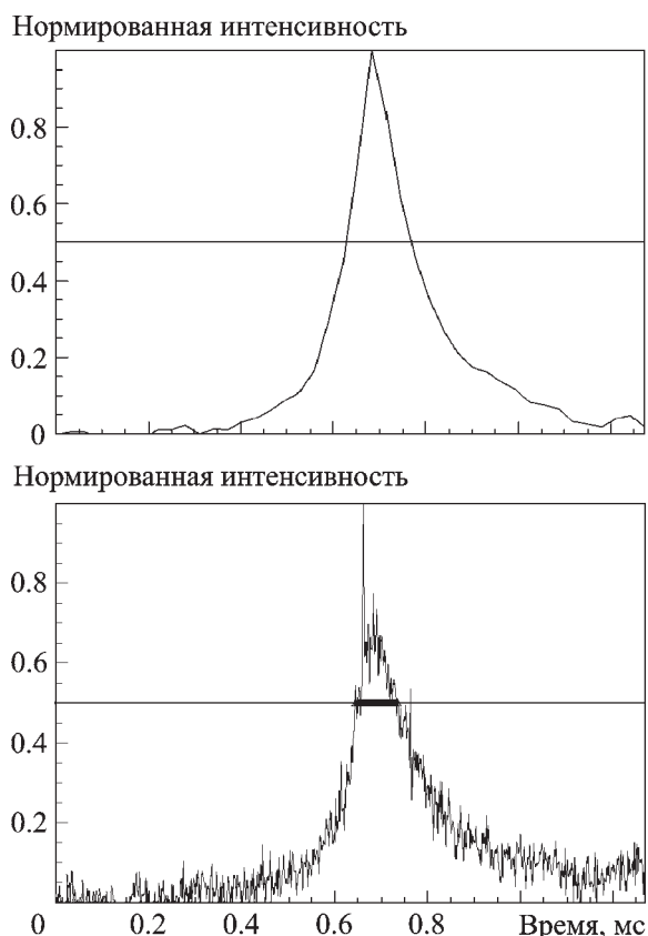
Рис. 5. Средний нормированный профиль субмиллисекундных структур SED при анализе с временным разрешением 31.5 мкс (верхняя панель) и 2 мкс (нижняя панель). Горизонтальной линией обозначен уровень половины максимума интенсивности вспышки
