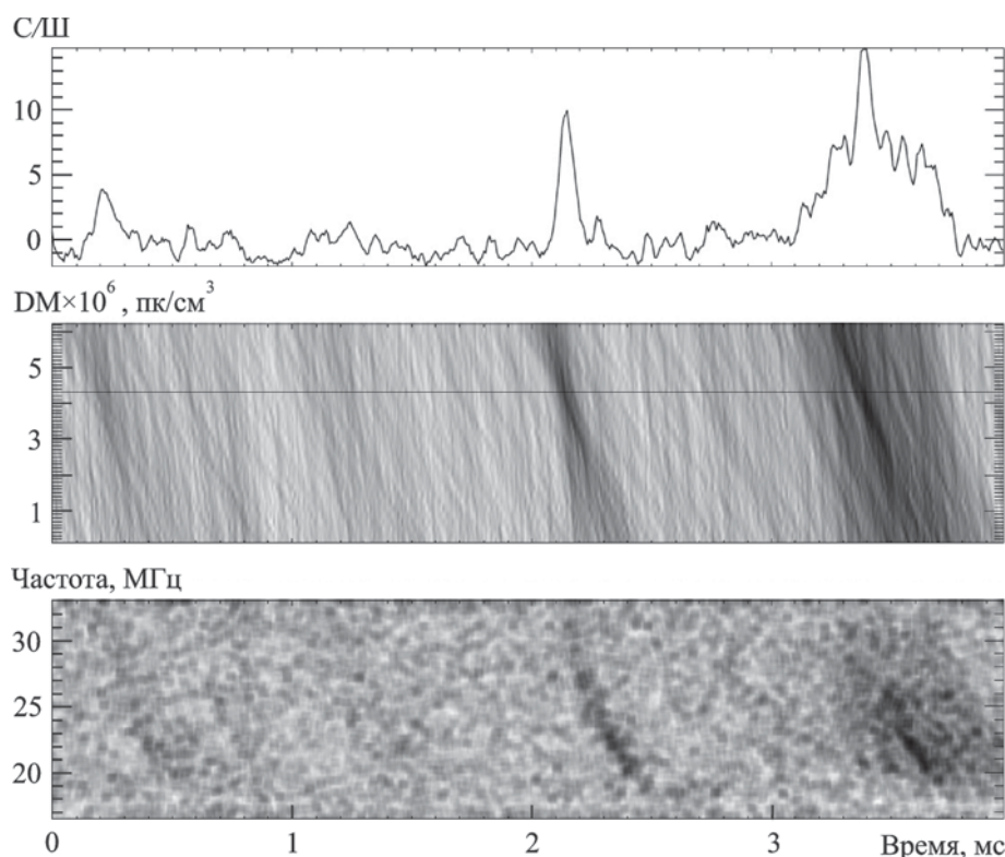
Рис. 2. Участок записи динамического спектра, содержащий молнию (нижняя панель), зависимость соотношения С/Ш от DM (средняя панель) и профиль накопленного по частоте сигнала в полосе 16.5 ÷ 33 МГц (верхняя панель)
