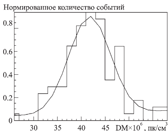
Рис. 3. Гистограмма распределения молний по значениям DM. Сплошной кривой показана аппроксимация полученного распределения комбинацией функции Гаусса и квадратичной функции
