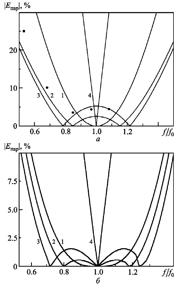
Рис. 8. Частотные зависимости паразитной составляющей на выходе широкополосной полуволновой ДФС, работающей в поле линейно поляризованной волны (а) и в поле кругополяризованной волны (б) при различных углах разворота средней ДЭ: \varphi = 60^\circ – кривая 1, \varphi = 59^\circ – кривая 2, \varphi = 58^\circ – кривая 3. Для сравнения представлена аналогичная зависимость для обычной полуволновой ДФС (кривая 4). Точками отмечены экспериментально измеренные значения амплитуды паразитного сигнала
