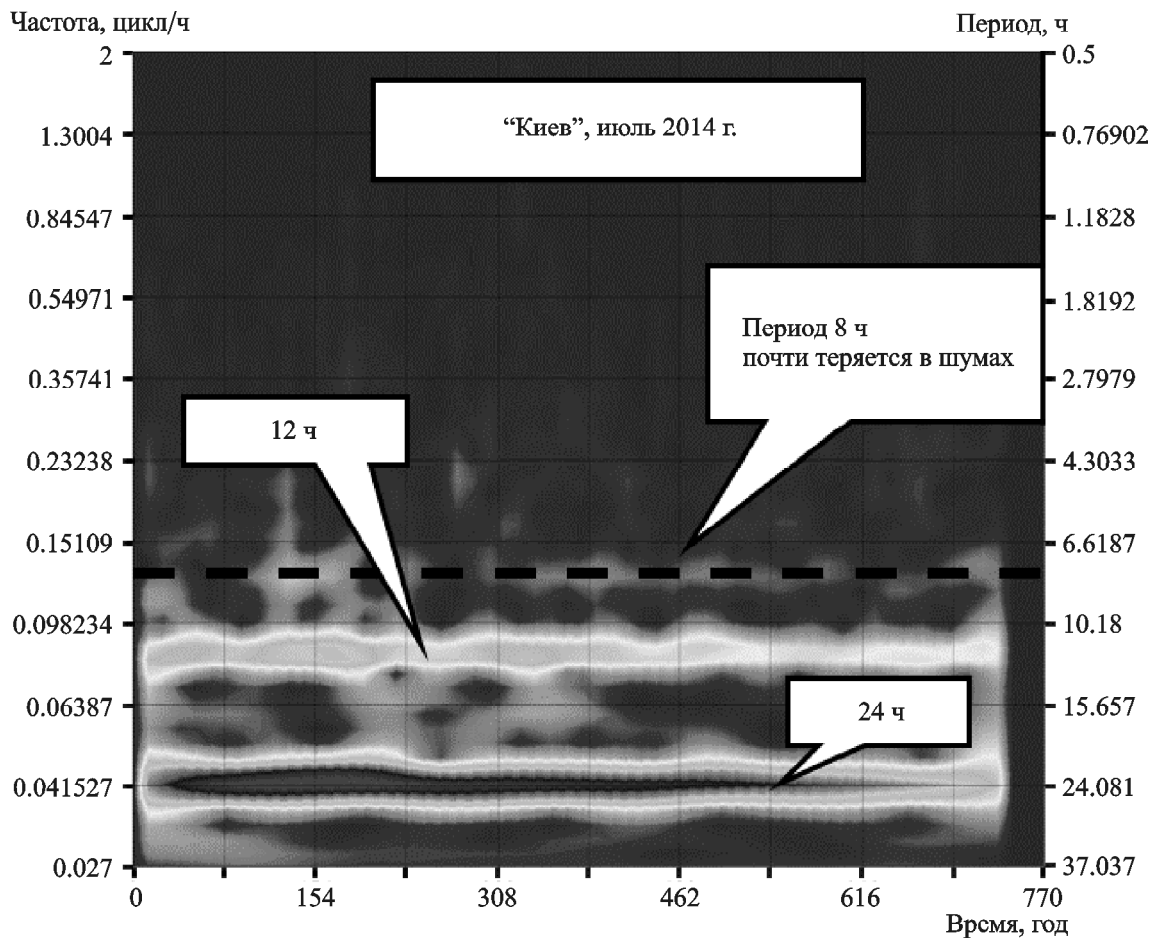
Рис. 5. Пример ослабления быстрых вариаций с периодом меньше 12 ч (по данным ГО “Киев”, зарегистрированным в июле 2014 г.)
