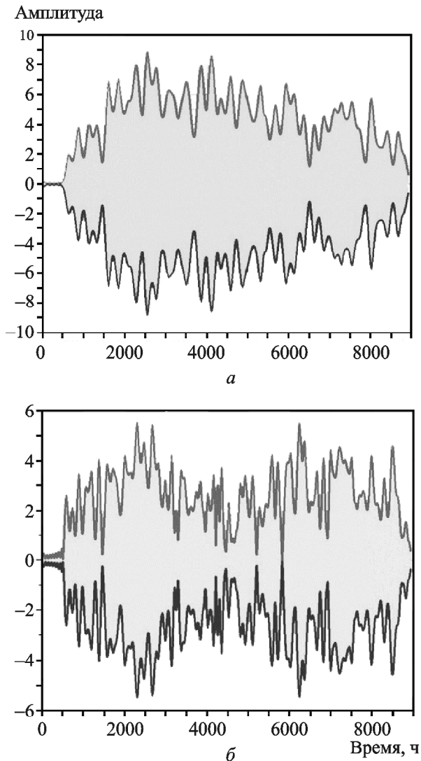
Рис. 4. Пример представления отдельных квазигармонических колебаний с периодами \approx 12 ч (а) и 8 ч (б) с амплитудной модуляцией, выделенных методом фурье-фильтрации (ГО “Одесса”, 2015 г.)
