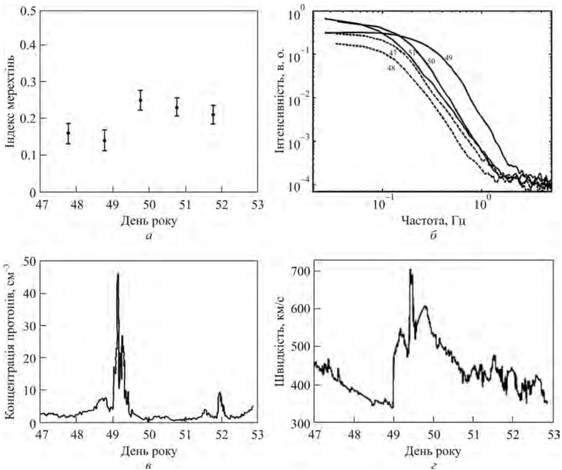
Рис. 7. Індеси (а) і спектри (б) мерехтін, отримані методом міжпланетних мерехтін (радіотелескоп УТР-2), та зміни концентрації протонів (в) і швидкості сонячного вітру (г), виміряні на орбіті Землі космічним апаратом Wind. Дані космічного апарата Wind взяті з бази даних OMNI NASA/GSFC на сторінці OMNIWeb ( https://omniweb.gsfc.nasa.gov )
