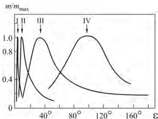
Рис. 2. Залежність індексу мерехтінь від елонгації та частоти спостережень: I – частота 2700 МГц (радіоджерело 3C279), II – 430 МГц (радіоджерело СТА-21), III – 74 МГц (радіоджерело 3C144) [3] та IV – 25 МГц (радіоджерело 3C144) [4]
