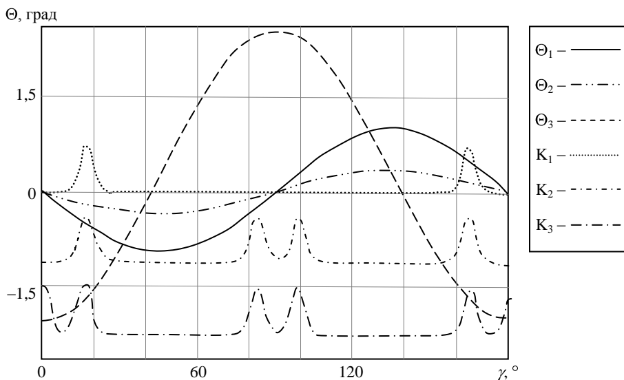
Рис. 2. Аналіз K в залежності від \gamma
