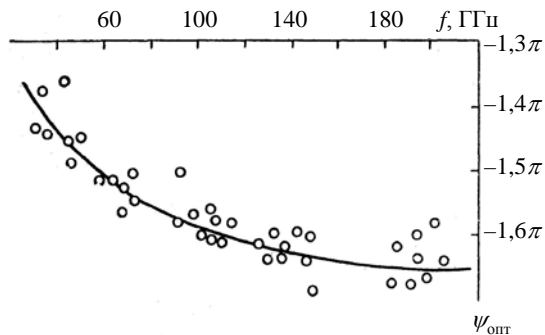
Рис. 3. Характер сдвига фазы 1-й отрицательной гармоники, соответствующей максимальному значению генерируемой мощности в области перестройки клинотрона, для клинотронов, генерирующих в диапазоне частот 35...220 ГГц
