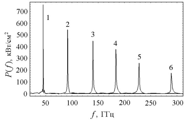
Рис. 8. Фурье-спектр плотности выходной мощности P(f) шести вариантов Si ЛГД в режиме когерентных двухчастотных автоколебаний
