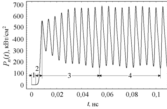
Рис. 7. Динамика развития и установления автоколебаний электронной компоненты плотности мгновенной мощности P_n(t) когерентного Si ЛГД
