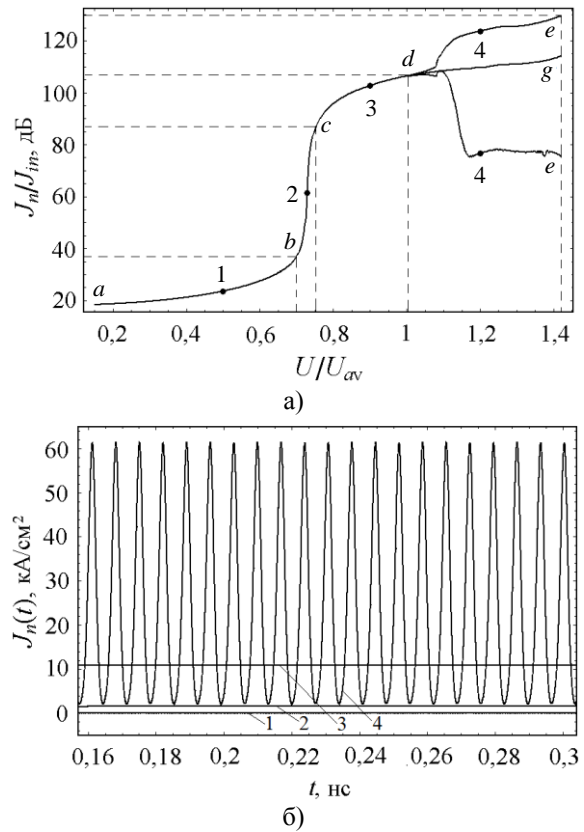
Рис. 1. Статическая ВАХ ЛГД на основе резкого GaAs p - n -перехода (а) и зависимость от времени электронной компоненты плотности лавинного тока J_n(t) в различных точках ВАХ (б). Кривые 1-4 соответствуют точкам 1-4 ВАХ
