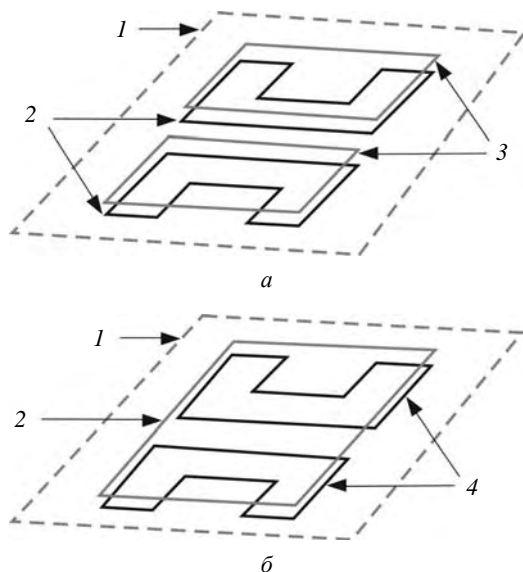
Рис. 2. Моделирование плоскостного сочленения канала Флоке (1) и волноводных каналов (2) сложного поперечного сечения с использованием: a – индивидуальных «виртуальных» волноводов (3); б – общего «виртуального» волновода (4)
