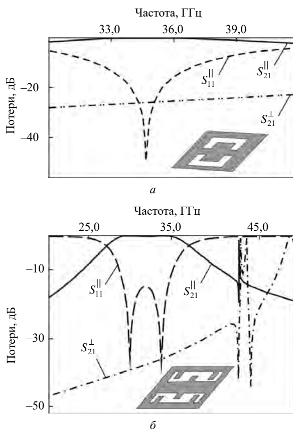
Рис. 3. Частотные характеристики вносимых и обратных потерь: a – одиночной решетки с парой П-образных щелей на элементарном периоде (угол падения \theta = 8^\circ ); б – сдвоенной решетки с парой меандроподобных щелей на элементарном периоде (нормальное падение)
