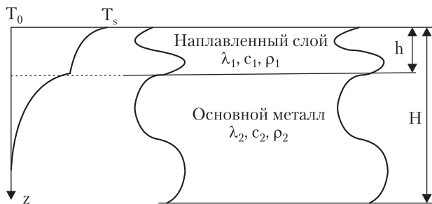
Рис. 2. Схема распределения температур T(z, t) по глубине z направляемого слоя и основного металла (подложки) при лазерной наплавке
