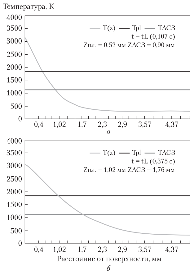
Рис. 6. Распределение температуры по глубине при лазерной наплавке сплава на основе никеля с содержанием хрома в пределах 8 \div 16\% на низколегированную сталь (20ХН): a – распределение T(z, 0,107) при P = 2,5 кВт, V = 100 м/ч, d_{II} = 3 мм; b – распределение T(z, 0,375) при P = 1,5 кВт, V = 29 м/ч, d_{II} = 3 мм
