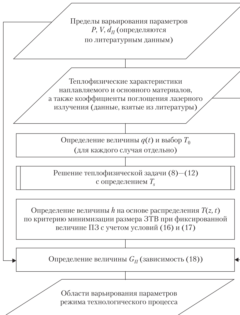
Рис. 5. Алгоритм расчетного определения технологических режимов лазерной наплавки
