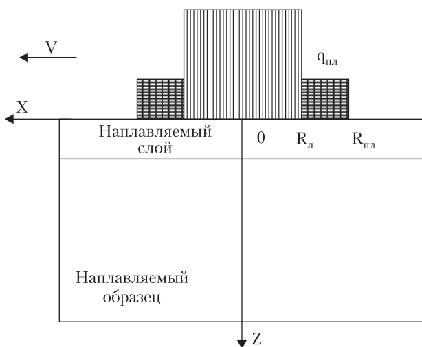
Рис. 3. Схема распределения тепловых потоков от лазерного q_l (радиусом R_l = d_{пл}/2 ) и плазменного q_{пл} (радиусом R_{пл} ) источников тепла при комбинированной лазерно-плазменной наплавке
