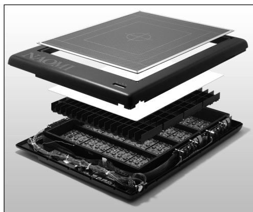
Рис. 3. Конструкция 192-сенсорной панели NAOMI, по-слою сверху—вниз: дека, преобразующий экран, бленды с объективами, поле сенсоров с электроникой
