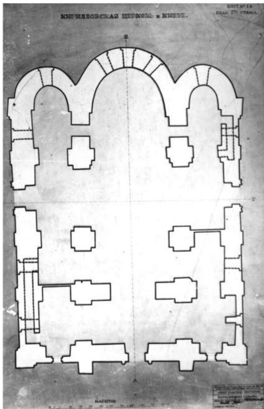
Рис. 18. План церкви з позначенням перегородок, створених у XIX ст. Фото 1930-х рр.
