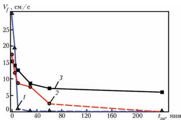
Рис. 3. Зависимость скорости распространения фронта реакции СВС ( V_f ) для многослойных фольг Al_{75}Ni_{25} с разным периодом чередования слоев ( \lambda ) от времени старения ( t_{ag} ) при температуре 250 °С (штриховые линии обозначают прекращение инициации реакции СВС): 1 — \lambda = 60 ; 2 — 160; 3 — 520 нм
