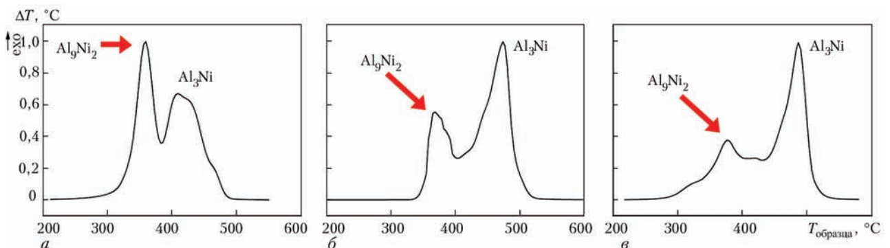
Рис. 5. Нормированные на максимум термограммы многослойных фольг Al/Ni ( Al_{75}Ni_{25} ) с периодом чередования слоев 120 (а), 200 (б) и 440 нм (в). Стрелкой указан экзотермический пик, соответствующий формированию фазы Al_9Ni_2
