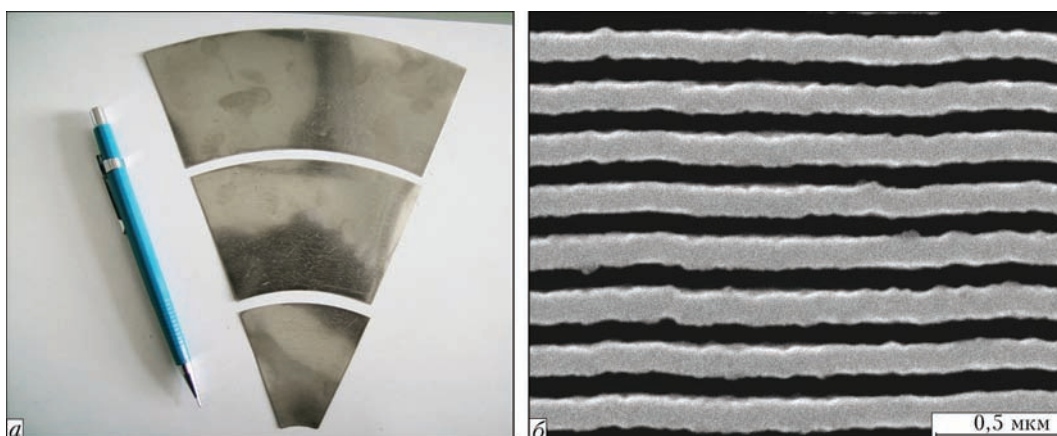
Рис. 2. Внешний вид одного из секторов многослойной Al/Ni фольги (а) и характерное электронно-микроскопическое изображение ее поперечного сечения (б)
