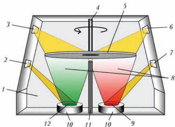
Рис. 1. Схема установки для послойного электронно-лучевого осаждения: 1 — рабочая камера; 2, 7 — электронно-лучевые пушки испарителей № 1 и 2 соответственно; 3, 6 — электронно-лучевые пушки нагревателей № 1 и 2 соответственно; 4 — держатель подложки; 5 — вращающаяся подложка; 8 — паровые потоки; 9, 12 — слитки алюминия и никеля соответственно; 10 — водоохлаждаемые тигли; 11 — непроницаемый экран
