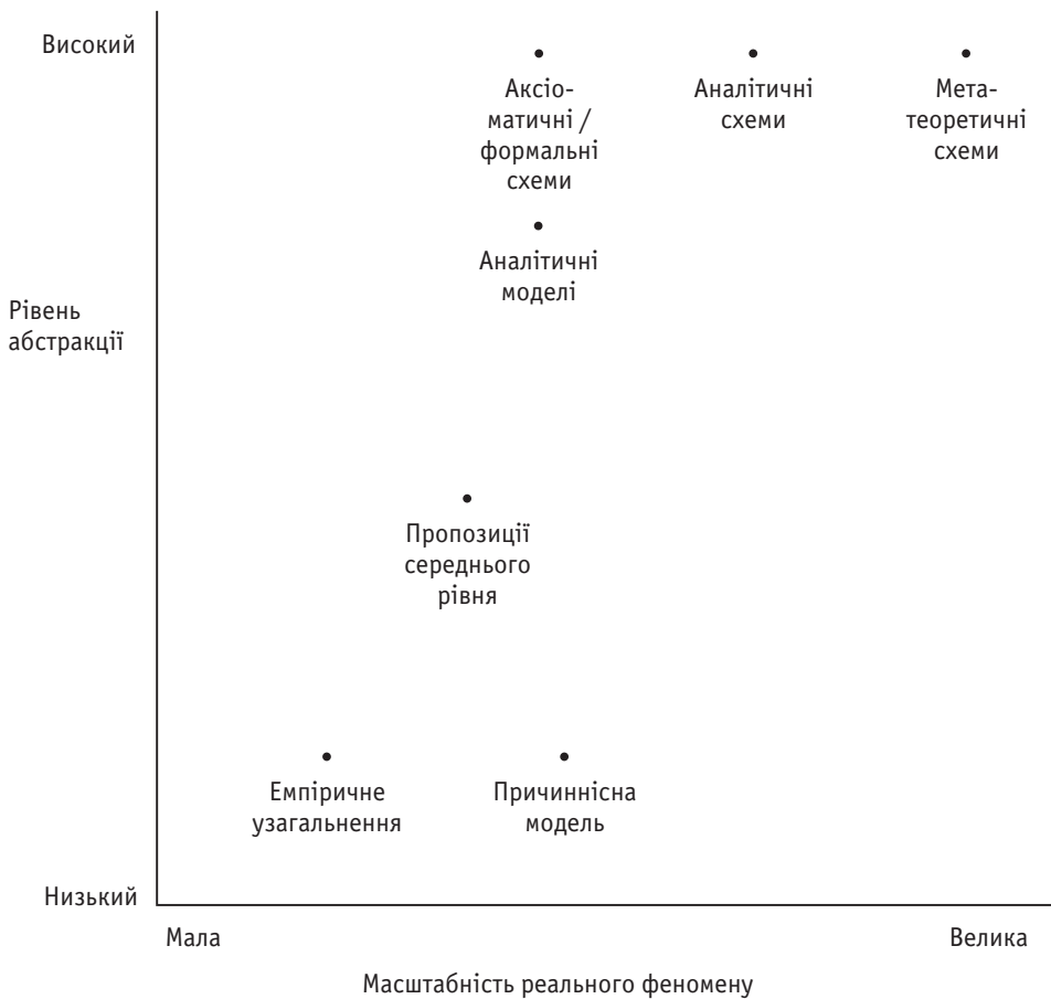
Рис. 4. Варіації у типах теоретичних форматів [Turner, 1990b: p. 21]
