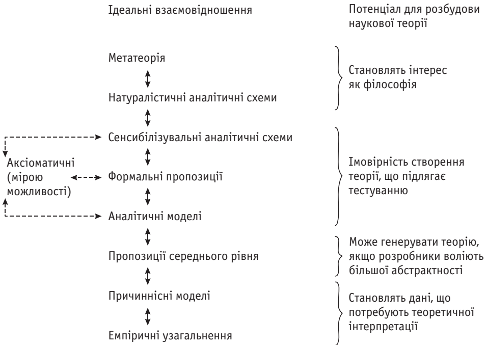
Рис. 5. Взаємовідношення між теоретичними підходами і потенціалом розбудови теорії [Turner, 1990b: р. 26]
