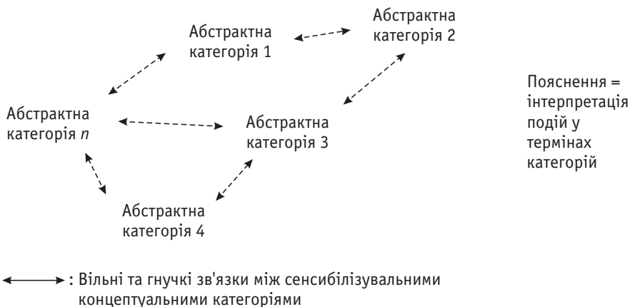
Рис. 3. Типи аналітичних схем [Turner, 1990b: p. 10]
