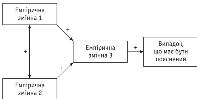
Рис. 2. Типи схем моделювання [Turner, 1990b: р. 19]
