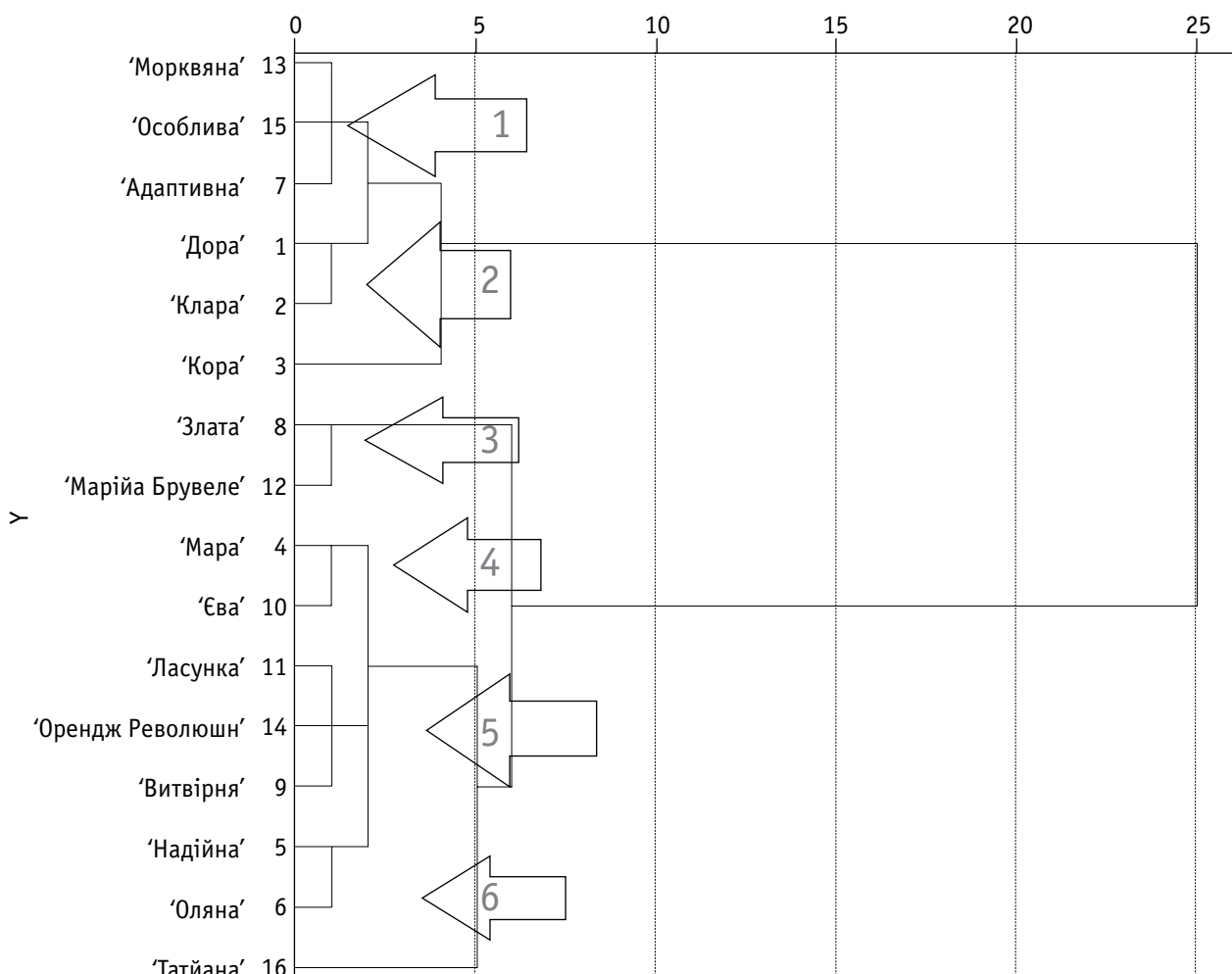
Рис. 2. Дендрограма результатів кластеризації сортів обліпихи крушиноподібної з використанням методу Варда
