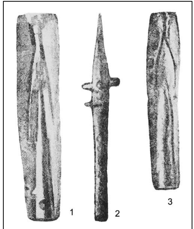
Рис. 1. Ливарні форми із збірки Національного музею історії України: 1-2 – колекція Б.І. Ханенка (с. Букрин); 3 – колекція О.О. Бобринського (м. Сміла?)
