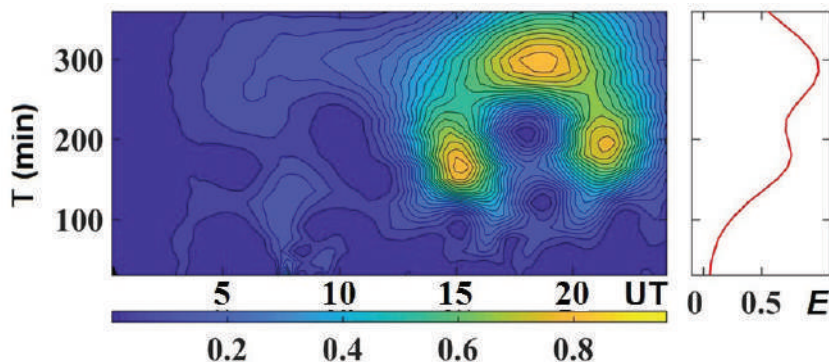
Рис. 4. Результати спектрального аналізу за допомогою АПФ для 14 листопада 2012 р. Праворуч показані відповідні енергограми. Fig. 4. Results of spectral analysis using the adaptive Fourier transform for November 14, 2012. The corresponding energygrams are given on the right.
