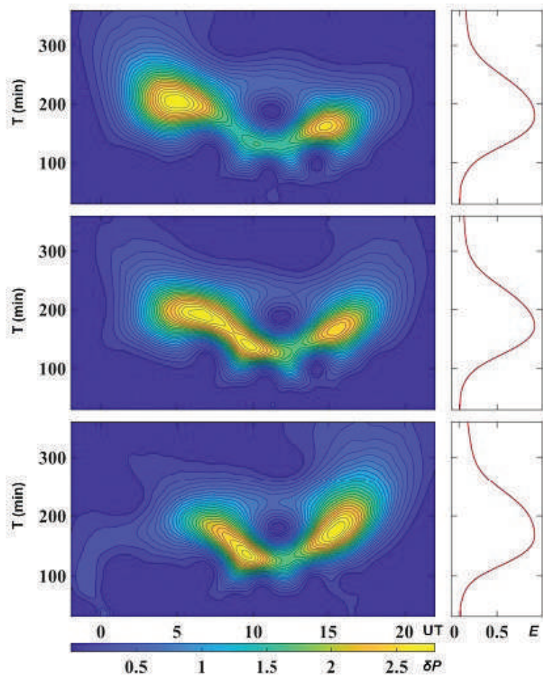
Рис. 8. Те ж, що й на рис.6, для 15 листопада 2012 р. і діапазону періодів 30 – 360 хв. Fig. 8. Same as in Fig. 6, for November 15, 2012 and the period range of 30 - 360 min.
