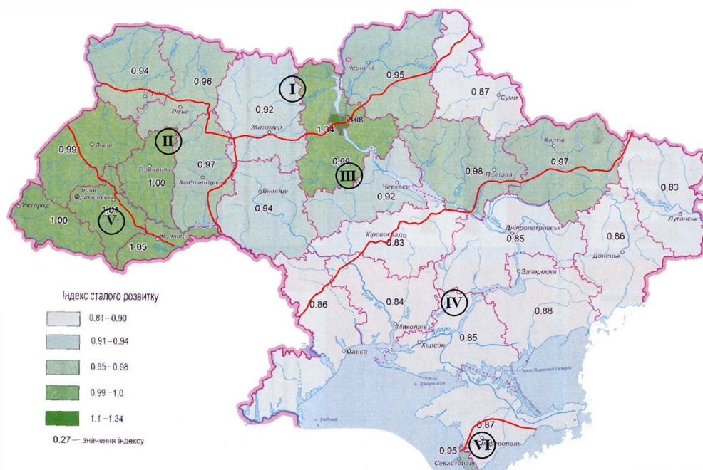
Рис. 6.8. Індекс сталого розвитку України за 2013 р. (за М. З. Згуровським): I — зона мішаних (хвойно-широколистяних) лісів; II — зона широколистяних лісів; III — лісостепова зона; IV — степова зона; V — регіон Карпат; VI — регіон Криму
