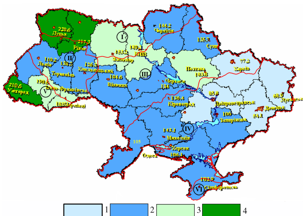
Рис. 6.9. Інтегрований індекс соціоприродного розвитку регіонів України за 2012 р. (за даними ЦАКДЗ ІГН НАН України) 1 — 50–100; 2 — 100.01–150; 3 — 150.01–200; 4 — 200.01–250 I — зона мішаних (хвойно-широколистих) лісів; II — зона широколистих лісів; III — лісостепова зона; IV — степова зона; V — регіон Карпат; VI — регіон Криму
