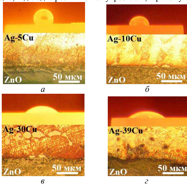
Рис. 2. Фотографії крапель срібло—мідь з різними концентраціями міді на поверхні ZnO-кераміки (1000 °С, 30 хв) та відповідні структури перехідних областей ( \times 400 ): a — Ag—5Cu; б — Ag—10Cu; в — Ag—30Cu; г — Ag—39Cu.
