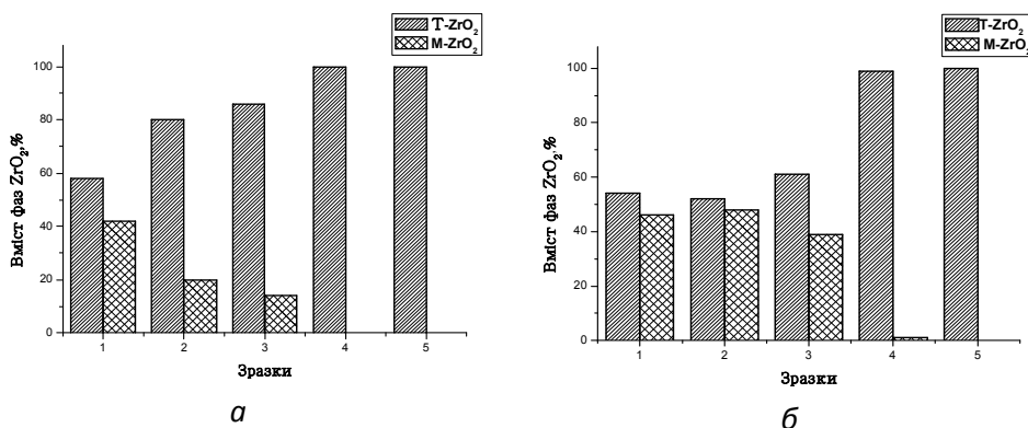
Рис. 2. Розподіл фаз у зразках Zr(3Y) (1), Zr(3Y2Ce) (2), Zr(2,5Y5Ce) (3), Zr(2Y8Ce) (4) та Zr(12Ce) (5) після обробки в гідротермальних умовах протягом 7 ( а ) та 14 год ( б ).
