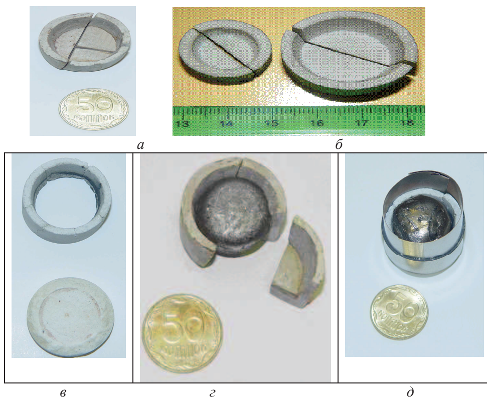
Рис. 3. Розбірні тиглі з фторидного вогнетриву: а — розбірний тигель з двох частин; б — розбірний тигель з трьох частин; в — розбірний тигель з чотирьох частин та окремо дно; г — сплав \text{Cu—15\% Nb} (плавлення при 1573 К) у розбірному тиглі; д — сплав \text{Cu—50\% Ti} (плавлення при 1423 К) у розбірному тиглі.
