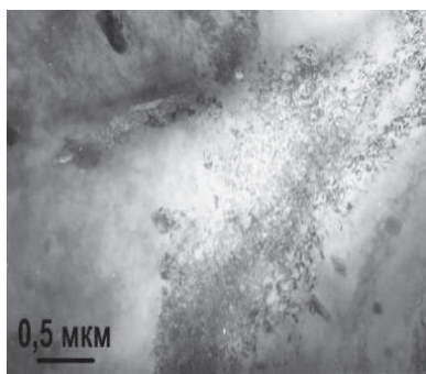
Рис. 6. Електронна мікроскопія про-деформованого на різні ступені дефор-мації сплаву АМг5: a — вихідний стан; б, в — \varepsilon = 2 та 10% відповідно.
