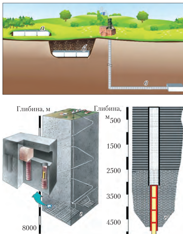
Рис. 1. Приклади концептуальних рішень сховищ для ізоляції різних класів РАВ [4, 5]: a — наземне сховище для ДНАВ; б — приповерхнє сховище для НАВ; в — підземне сховище геологічного типу на глибині до 700 м для САВ; z і z' — геологічне глибинне сховище для ВАВ — комбіноване шахтно-свердловинне ( z ) та свердловинне ( z' )
