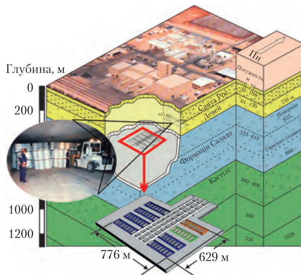
Рис. 3. Схема сховища геологічного типу WIPP у США для трансуранових відходів [6, 7]
