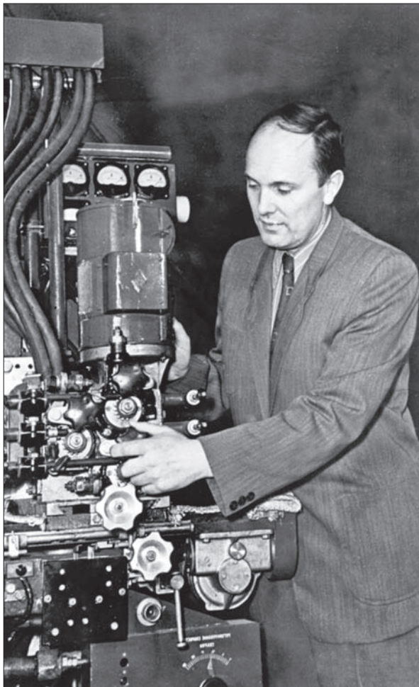
Борис Євгенович Патон біля автомата для електрошлакового зварювання, за створення якого йому присуджено Ленінську премію. Київ, травень 1957 р.
