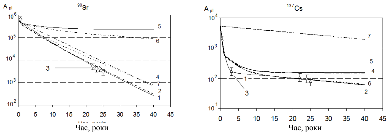
Рис. 1. Прогнозні оцінки вмісту радіонуклідів у багаторічних травах з контрастних за властивостями ґрунтів залежно від урахування основних процесів, які визначають динаміку накопичення радіонуклідів рослинами: ^{90}\text{Sr} , слабогумусований пісок: 1 - модель (1), ураховано всі фактори; 2 - модель (2), ураховано всі фактори; 3 - експериментальні дані; 4 - без урахування фізичного розпаду ^{90}\text{Sr} ; 5 - без урахування фізичного розпаду та виносу ^{90}\text{Sr} ; 6 - без урахування виносу ^{90}\text{Sr} ; 7 - без урахування динаміки вмісту рухливих форм ^{90}\text{Sr} . ^{137}\text{Cs} , чорнозем типовий важкосуглинний: 1 - модель (1), ураховано всі фактори; 2 - модель (2), ураховано всі фактори; 3 - експериментальні дані; 4 - без урахування фізичного розпаду ^{137}\text{Cs} ; 5 - без урахування фізичного розпаду та виносу ^{137}\text{Cs} ; 6 - без урахування виносу ^{137}\text{Cs} ; 7 - без урахування динаміки вмісту рухливих форм ^{137}\text{Cs} .
