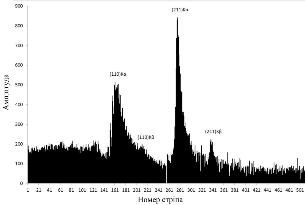
Рис. 4. Розподіл інтенсивності рентгенівських квантів у лінях (110)Ka та (211) Ka – фази ARMCO-заліза при кімнатній температурі, виміряний широкодіапазонною мікродетекторною системою в області малих кутів – лінія (110) – перша детекторна група: 1 - 256 каналів) та в області великих кутів – лінія (211) друга детекторна група: 257 - 512 каналів).
