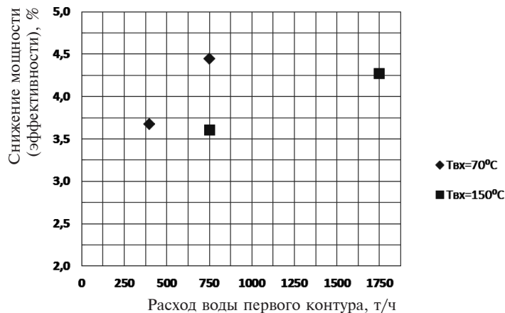
Рис. 10. Снижение мощности (эффективности) ТО CAO3 по сравнению с вариантом «чистого» ТО ( R = 10^{-5} \text{ м}^2 \cdot \text{К}/\text{Вт} )
