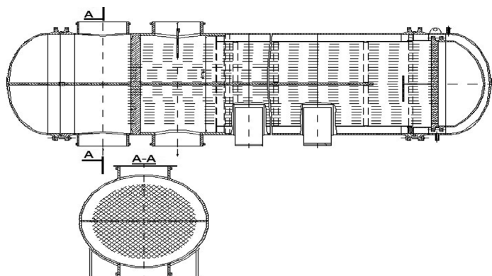
Рис. 1. Теплообменник аварийного и планового расхолаживания
