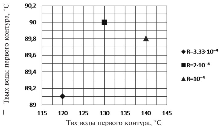
Рис. 6. Зависимость изменения температуры воды на выходе из ТО CAO3 от температуры на входе
