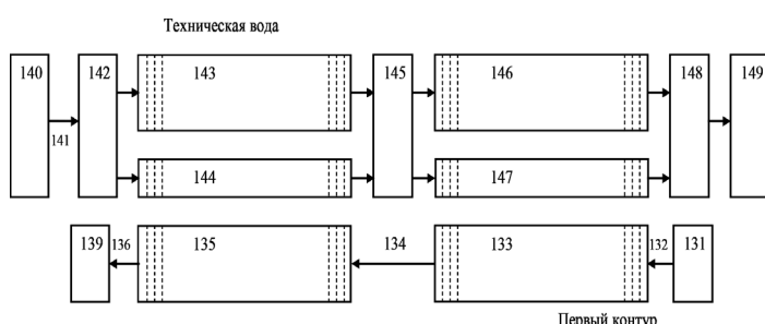
Рис. 2. Нодализация модели ТО САОЗ
