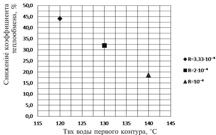
Рис. 8. Снижение коэффициента теплопередачи в зависимости от температуры воды на входе в ТО CAO3
