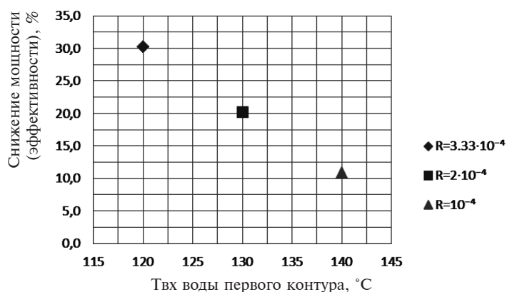
Рис. 7. Снижение мощности (эффективности) ТО CAO3 в зависимости от температуры на входе в ТО CAO3
