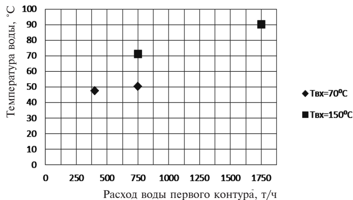
Рис. 9. Температура воды на выходе из ТО CAO3
