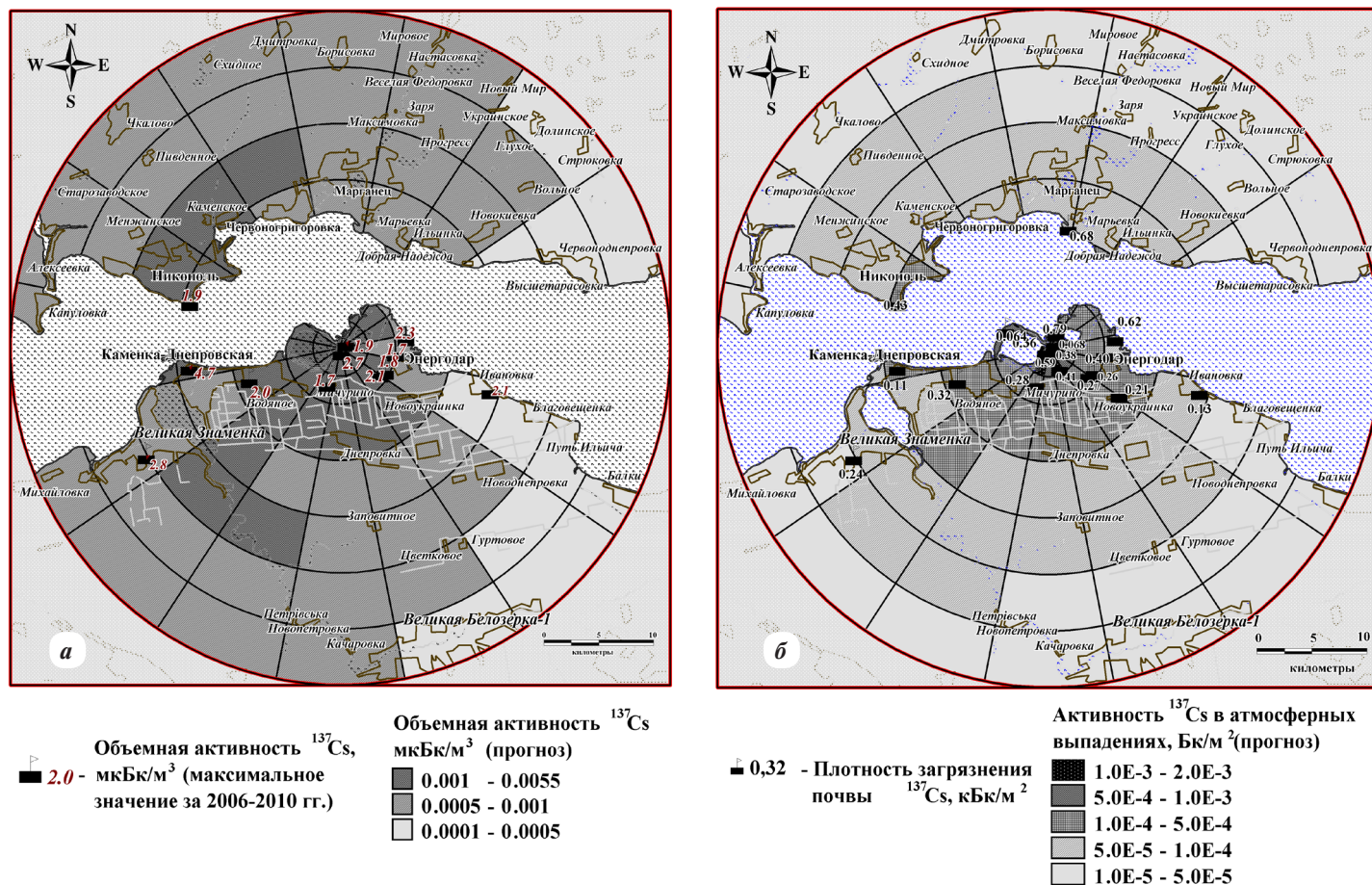
Рис. 1. Пространственное распределение расчетных значений объемной активности в приземном слое атмосферы (а) и атмосферных выпадений 137 Cs (б) на территории зоны наблюдения ЗАЭС, обусловленных газо-аэрозольными выбросами при штатном режиме эксплуатации КП РАО
