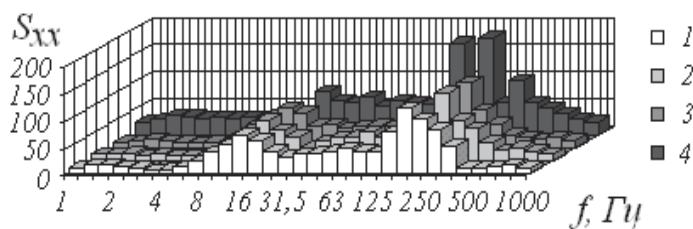
Рис. 6. Сопоставление частотной структуры АСП акустического шума в режиме начала кипения воды (параметры процесса: p=6,86 МПа, \rho_w=2450 кг/(м 2 .с); \Delta T_{\text{вых}}=14 К) в каналах различной геометрии:
