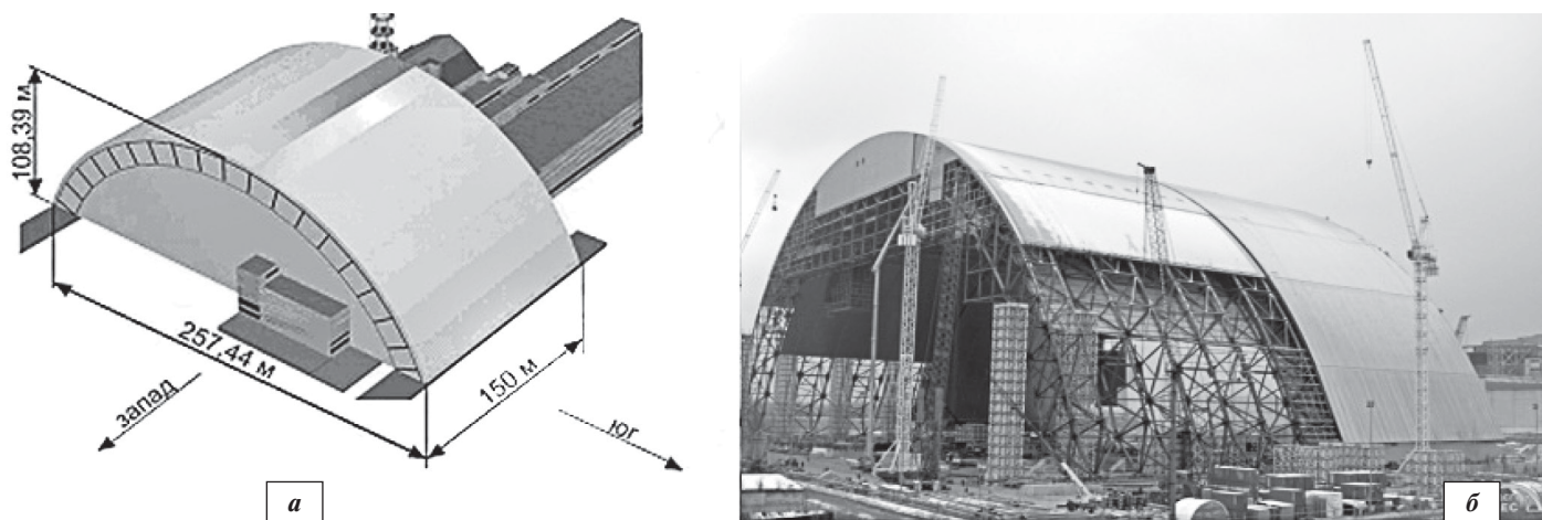
Рис. 3. Новий безпечний конфайнмент: а — проєктні розміри; б — монтаж арки на промайданчику ОУ
