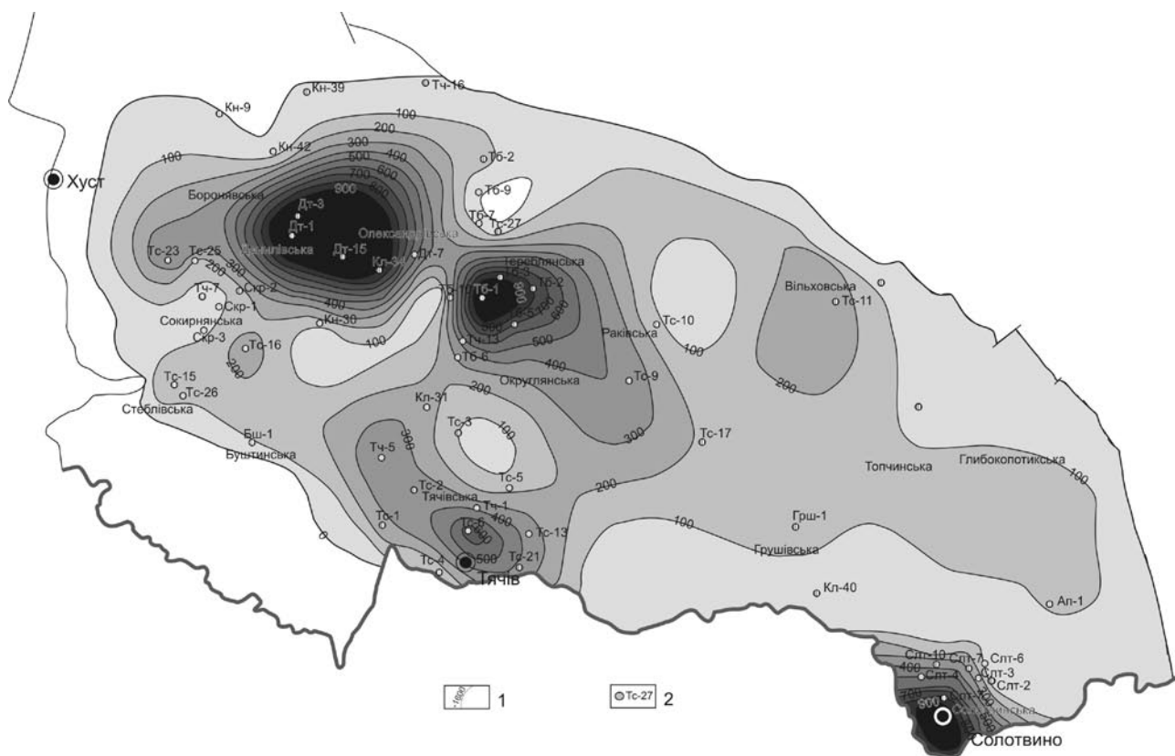
Рис. 1. Модель потужності соленої формації галотектокінетичного типу Закарпатського прогину 1 — ізолінії потужності соленої формації; 2 — свердловини
