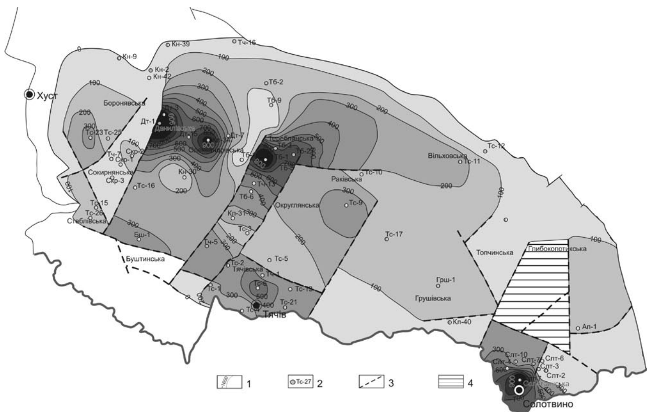
Рис. 2. Модель потужності соленої формації галотектокінетичного типу Закарпатського прогину з урахуванням розривних порушень 1 — ізолінії потужності соленої формації; 2 — свердловини; 3 — розривні порушення; 4 — малоінформативні ділянки
