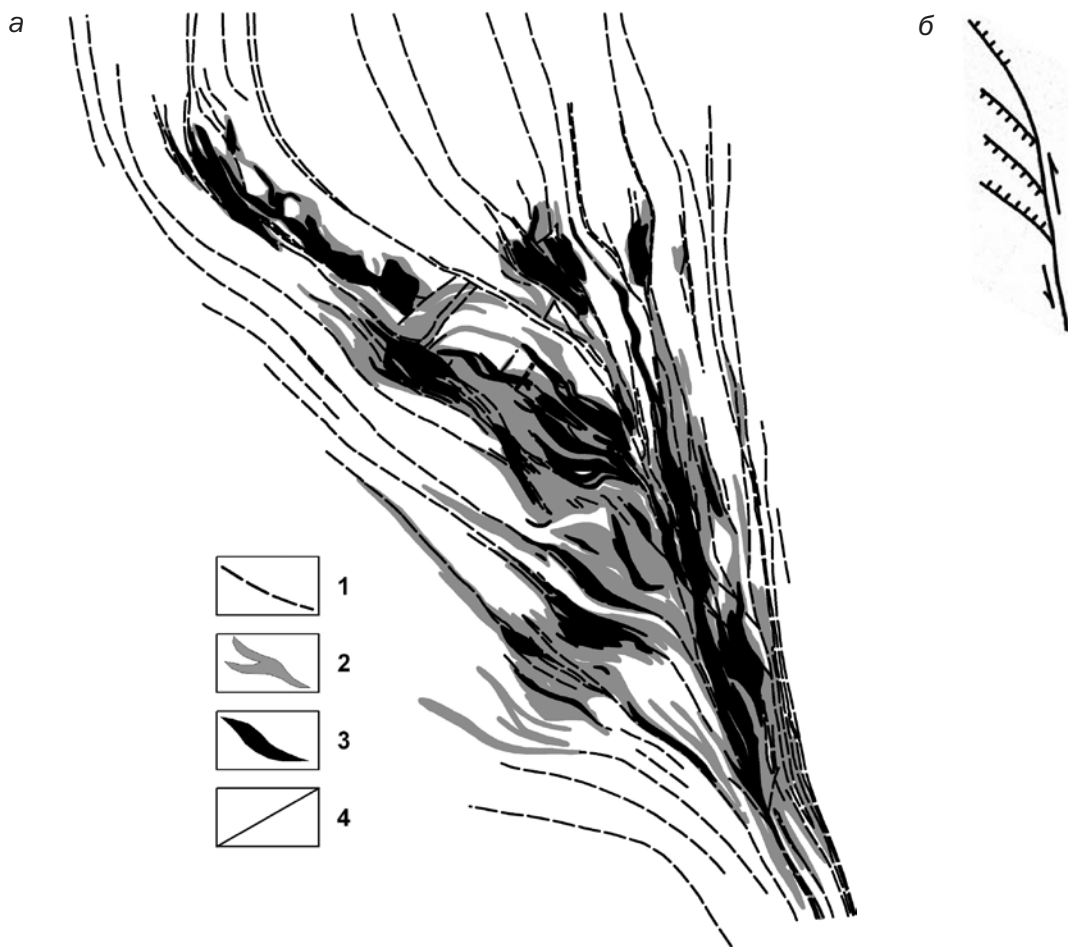
Рис. 2. Аналогія структурного рисунка Мічуринського родовища з типовим здвиговим структурним рисунком а) погоризонтний план Мічуринського родовища (на основі матеріалів м-бу 1:1.000, А.К. Прусс, 1967), 1 — розломи; 2 — альбітити; 3 — рудні тіла. б) структурний рисунок типу «кінський хвіст», за [14, 16]; зубчатою лінією позначено структури розтягування, стрілки показують напрямки здвигу
