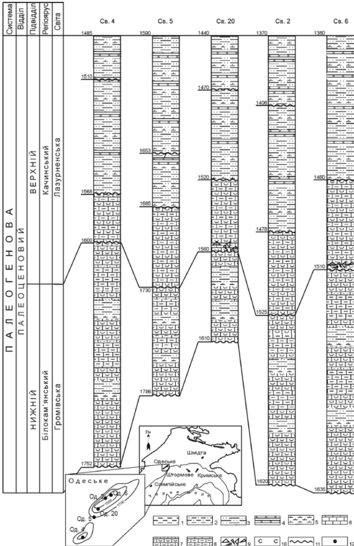
Рис. 2. Схема кореляції палеоценових відкладів підняття Одеське 1 — глини; 2 — глини алевритисті; 3 — алевроліти; 4 — пісковики; 5 — глини вапнисті; 6 — вапняки; 7 — вапняки органогенно-детритові; 8 — мергелі; 9 — брекчії; 10 — сидеритові породи; 11 — перерив; 12 — свердловина
