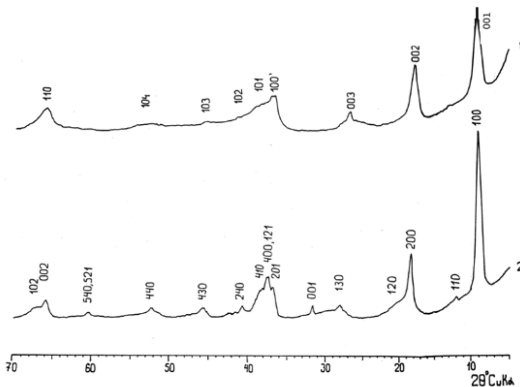
Рис. 1. Рентгенограммы 10 Å марганцевых минералов 1 — бузерит II, 2 — тодорокит
