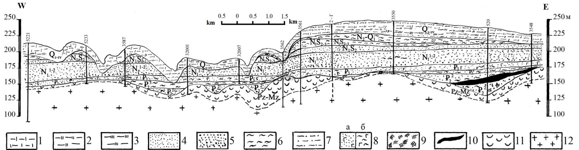
Рис. 2. Геологічний розріз осадового покриття Новокосянтинівського рудного поля та прилеглих територій по лінії I-I.
