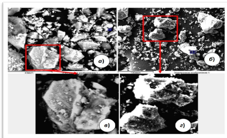
Рис. 1. Электронные фотографии проб продукта питания флотации без УЗВ (а) и после УЗВ (б), в, г – частица кварца в материале до и после УЗО Fig.1 Electronic photos of feed flotation samples before (a) and after the ultra sonic treatment (б), в, г – quartz particle in the material before and after ultra sonic treatment
