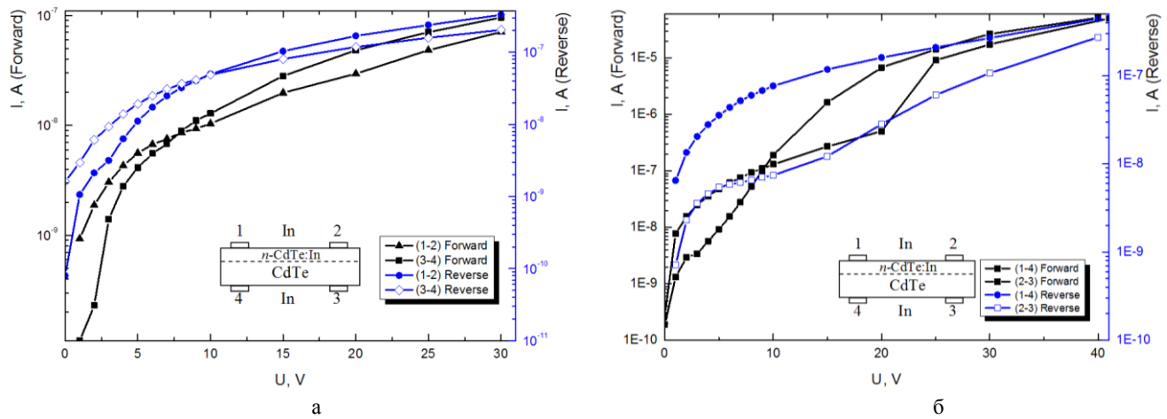
Рис. 3. Вольт-амперні характеристики структури In/CdTe/In. Fig. 3. The I-V characteristics of the In/CdTe/In structure.
